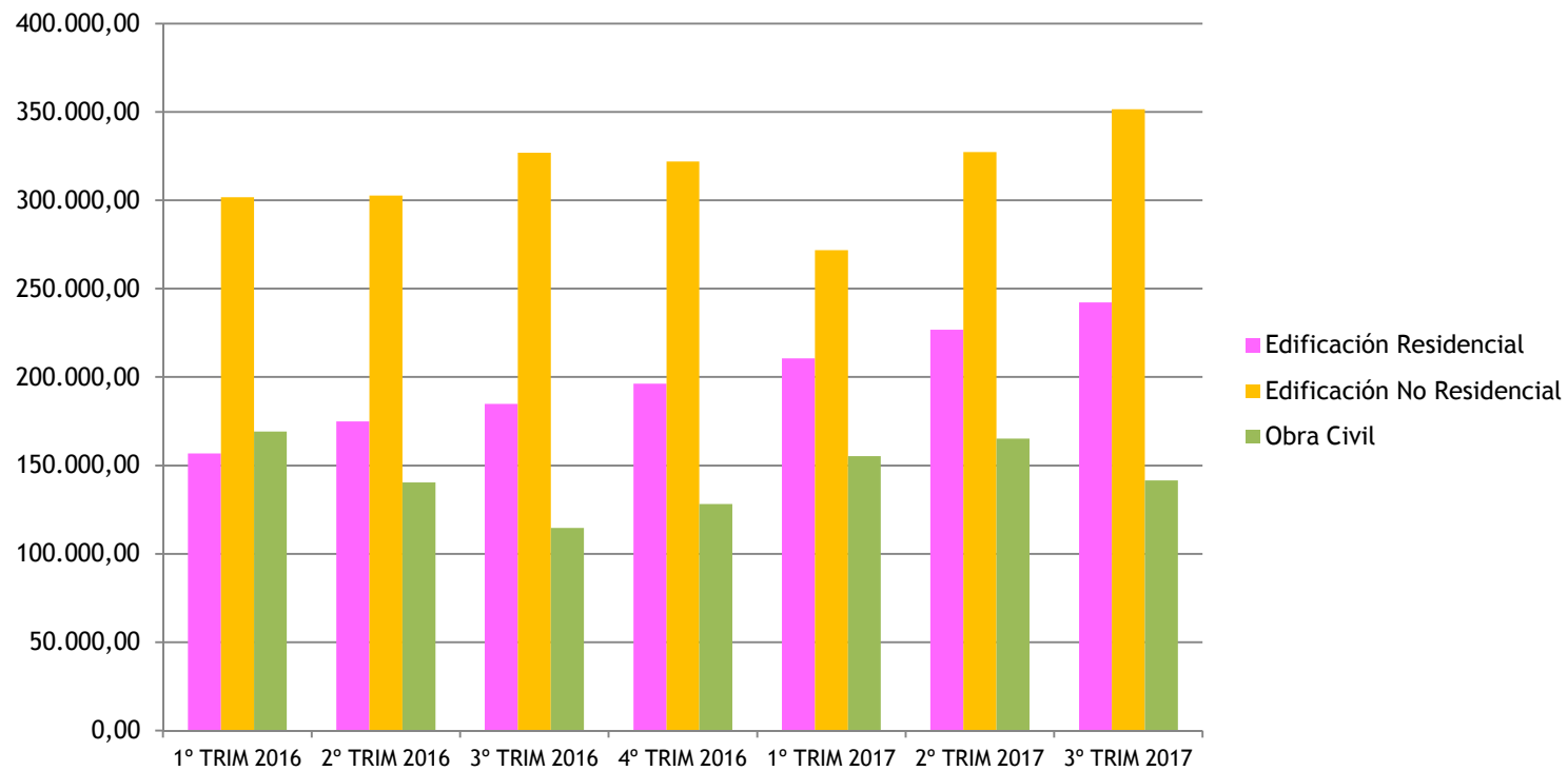
Consumo de Prefabricados de Hormigón. Por Tipos. OBRA NUEVA.
