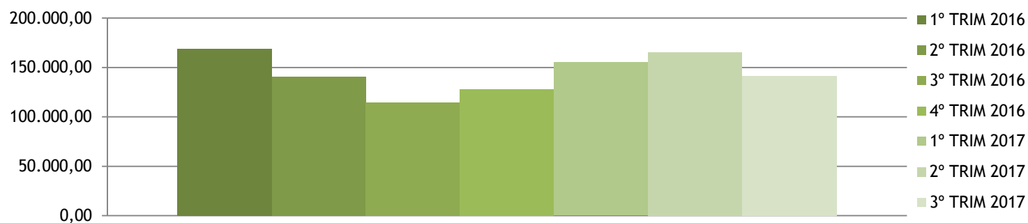
Consumo de Prefabricados de Hormigón. Obra Civil. Total. OBRA NUEVA.
