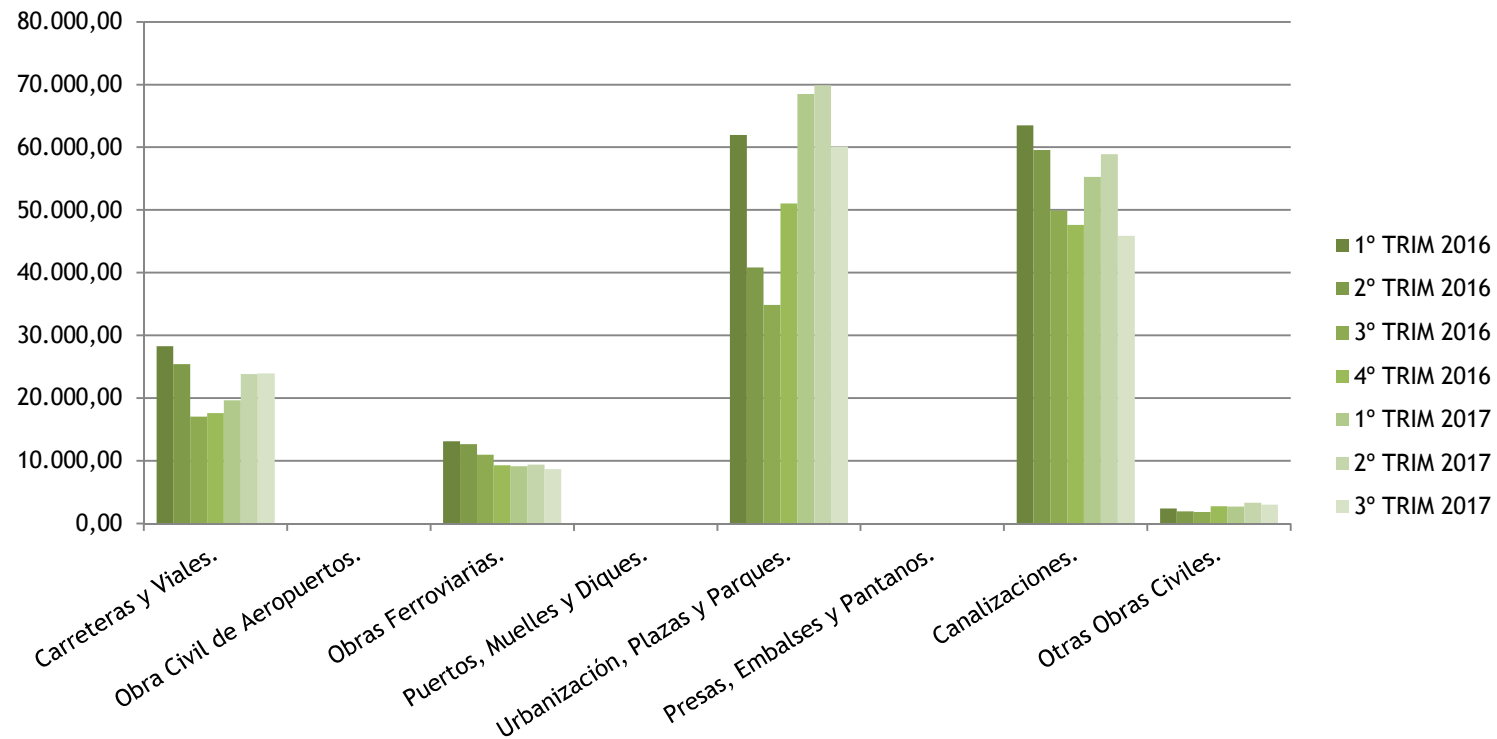
Consumo de Prefabricados de Hormigón. Obra Civil. Por Tipos. OBRA NUEVA.
